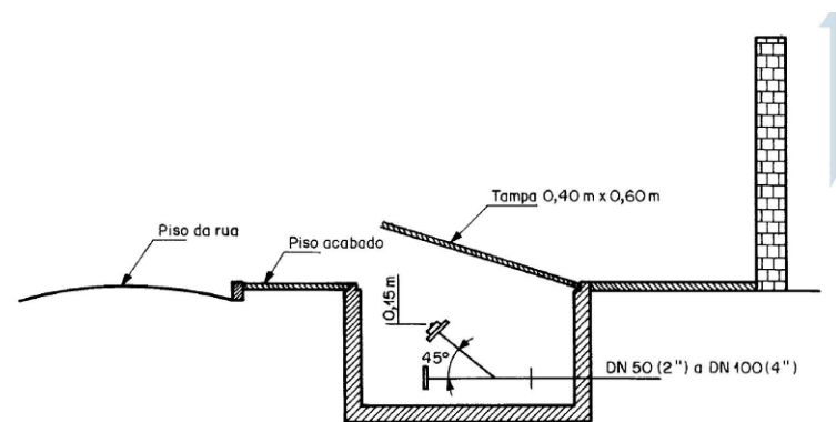
Figura 1 - Dispositivo de recalque no passeio
